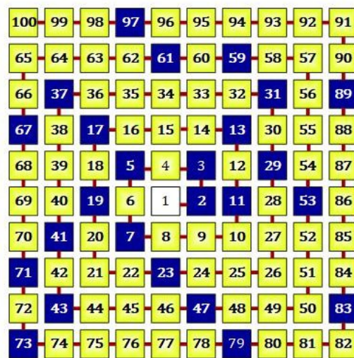
Abbildung 1: Die Ulam-Spirale
