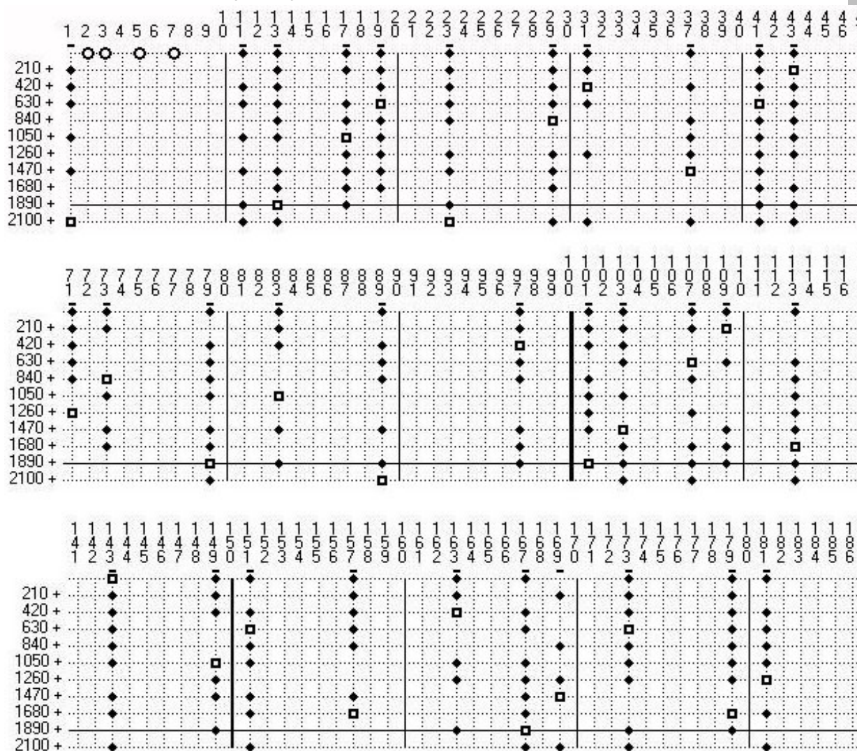
Abbildung 5: Der 210-er Stempel und die Primzahlen < 2310, angeordnet in Zeilen zu je 210 Spalten.
