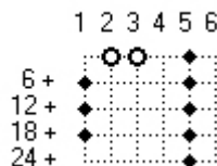
Abbildung 2: Der "6-er Stempel" und die Primzahlen &lt; 30, angeordnet in Zeilen zu je 6 Spalten
