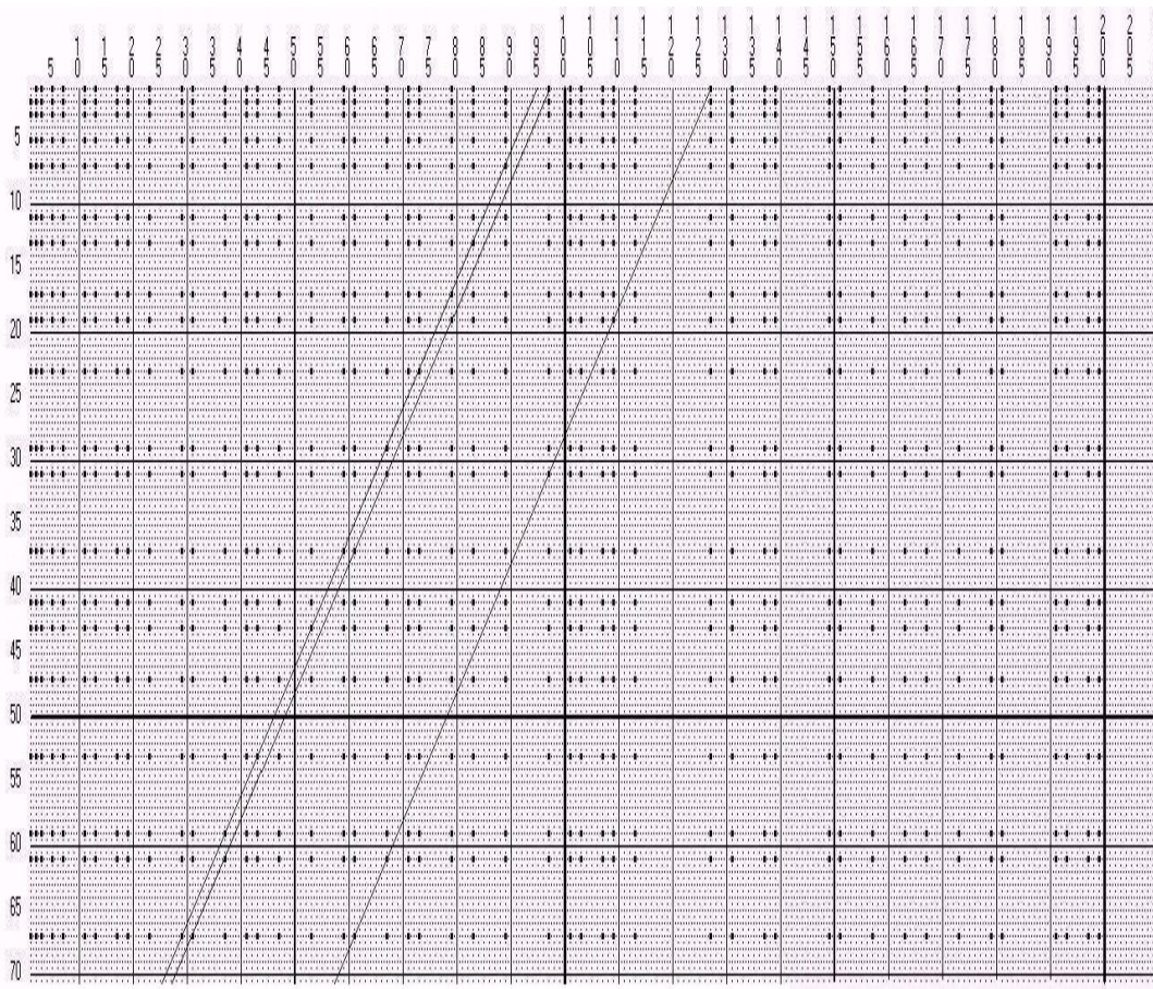
Abbildung 13: Startwert 97. Primzahlen und Modulo-Werte
