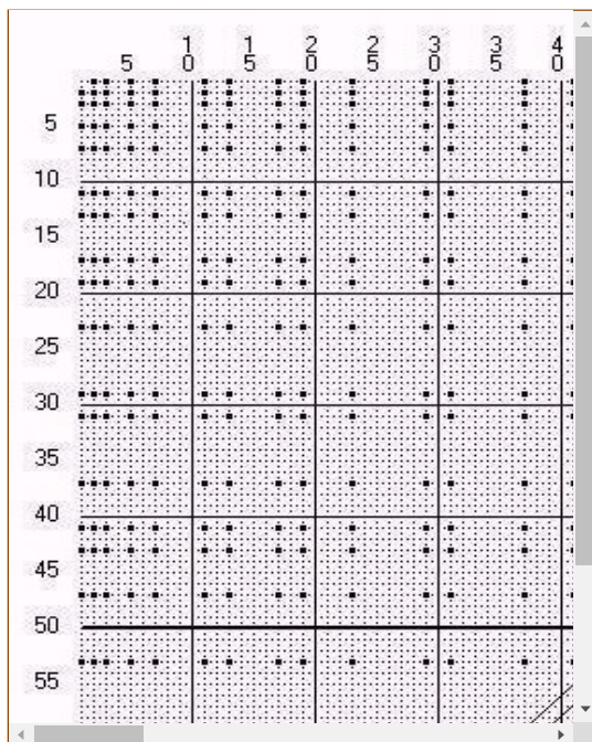
Abbildung 9: Primzahlen in waagrechter und senkrechter Darstellung
