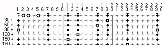
Abbildung 3: Der "30-er Stempel" und die Primzahlen &lt; 210, in Zeilen zu je 30 Spalten angeordnet.
